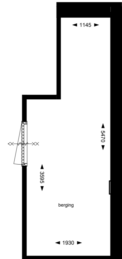
Externe berging eerste verdieping
