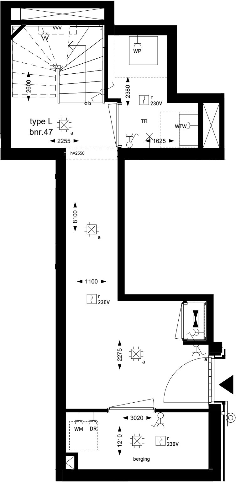
4e verdieping
