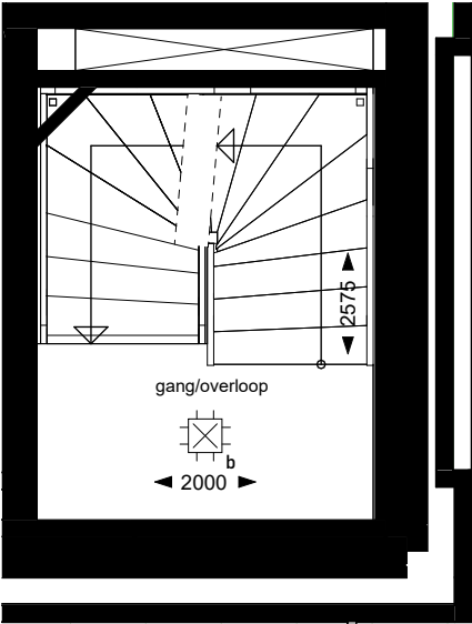
5e verdieping
